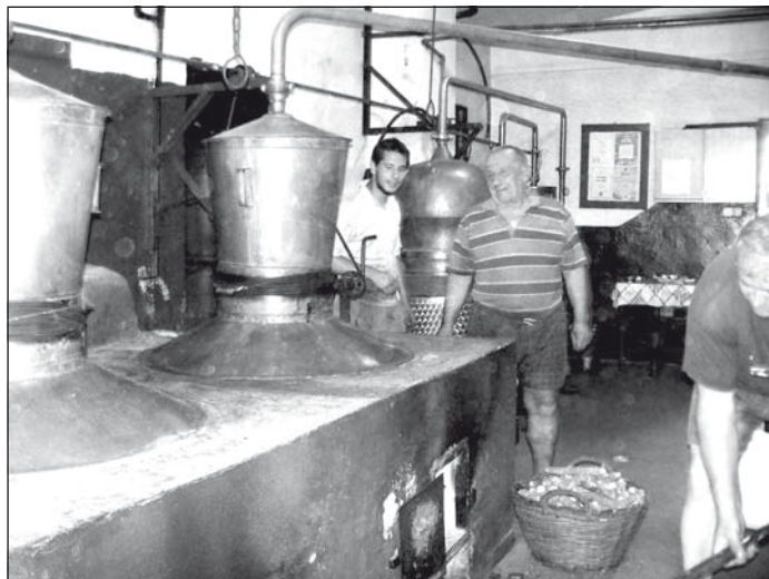
A Kohanecz bér-főzdében tornyos lepárlással készül a minőségi pálinka
